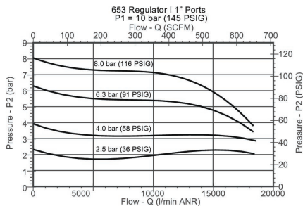
Diagrama de caudal G 1
