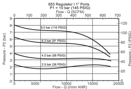
Diagramma della portata G 1
