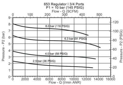
Diagramma della portata G 3/4
