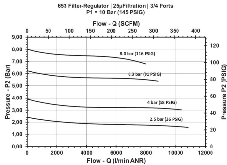
Diagramma della portata G 3/4
