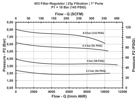
Diagramma della portata G 1
