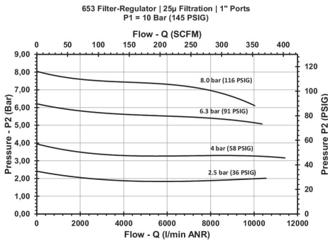
Diagrama de caudal G 1
