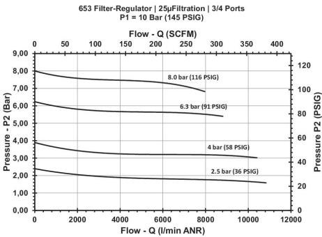
Diagrama de caudal G 3/4
