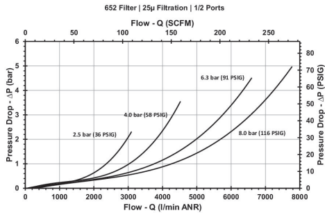
Diagramme du débit G 1/2
