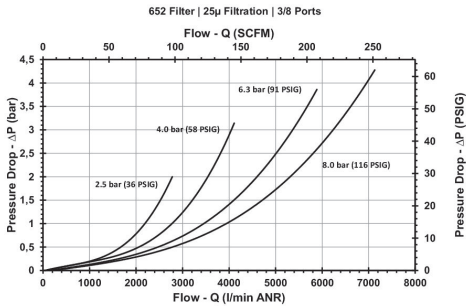
Diagramme du débit G 3/8
