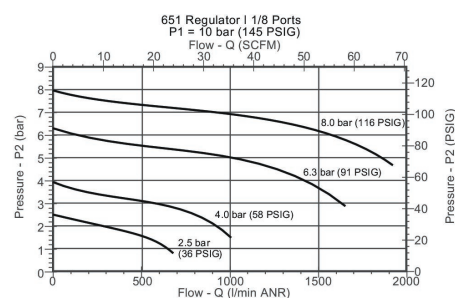
Diagrama de caudal G 1/8
