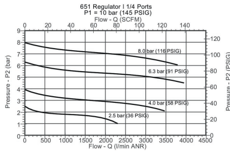
Diagramma della portata G 1/4
