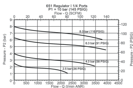
Diagramme du débit G 1/4
