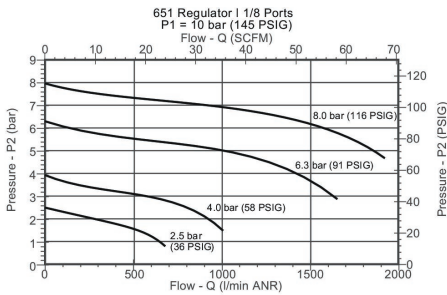
Diagramma della portata G 1/8
