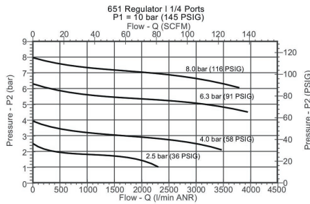
Diagrama de caudal G 1/4
