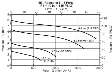
Diagramma della portata G 1/8
