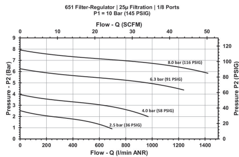
Diagramme du débit G 1/8
