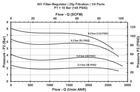
Diagramme du débit G 1/4
