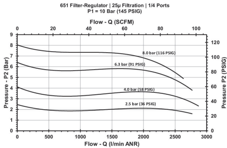
Diagrama de caudal G 1/4
