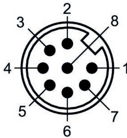
プラグのピン割り当て
