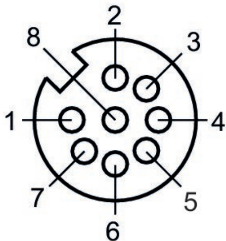
ピン割り当て、ソケット
