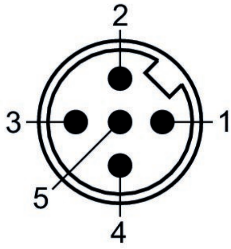
Polbild Stecker
