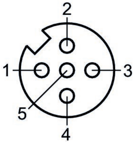
Polbild Buchse
