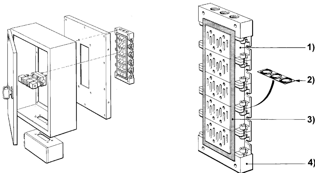
1) piastra intermedia 2) guarnizione piastra intermedia 3) listello di tenuta 4) piastra terminale
