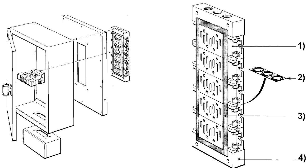
1) Plaque intermédiaire 2) Joint de plaque intermédiaire 3) Barre d'étanchéité 4) Plaque terminale
