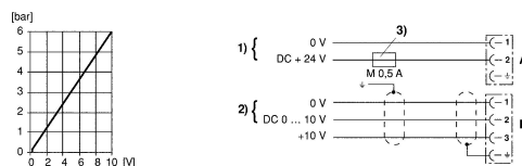
1) 供給電圧 2) 電圧制御 3) 供給電圧は外部ヒューズM 0.5 Aで保護します。EMVを確実にするためにプラグ2はスクリーンケーブルで接続します。A) プラグ1 B) プラグ2
