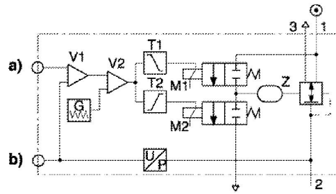
Schéma fonctionnel
