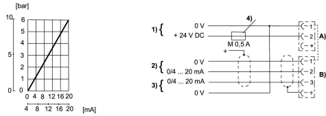
Fig. 1 Caratteristica e occupazione connettori per pilotaggio a corrente con uscita del valore effettivo
