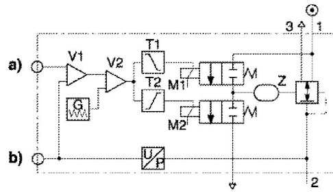
Schéma fonctionnel
