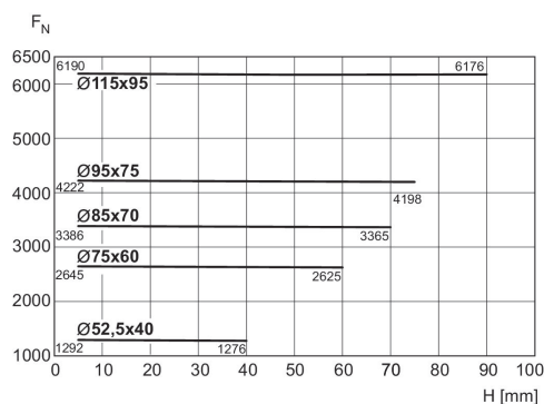
Curva característica de força/curso 6 bar
