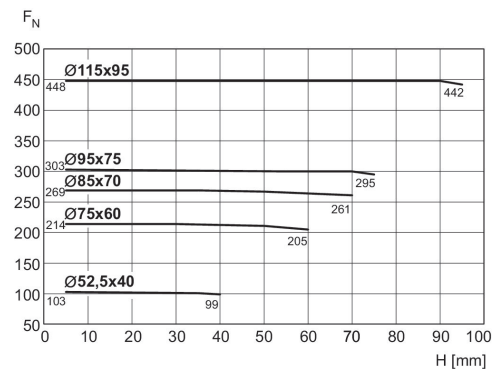
Courbe caractéristique force / course 0,5 bar
