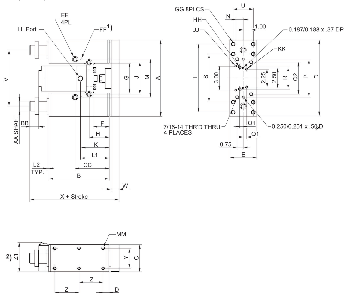
寸法 (インチ)
