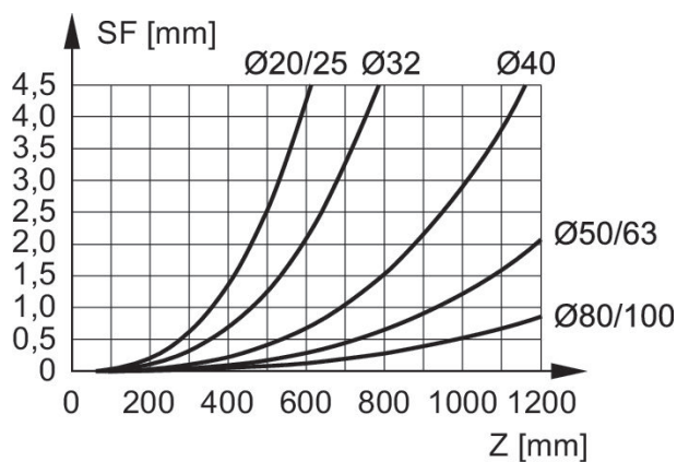
負荷10 Nによる曲がり
