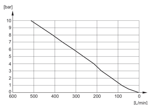
Durchflussdiagramm 1827430004
