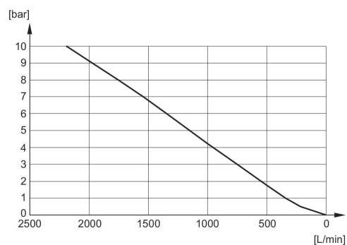
Durchflussdiagramm R412007876
