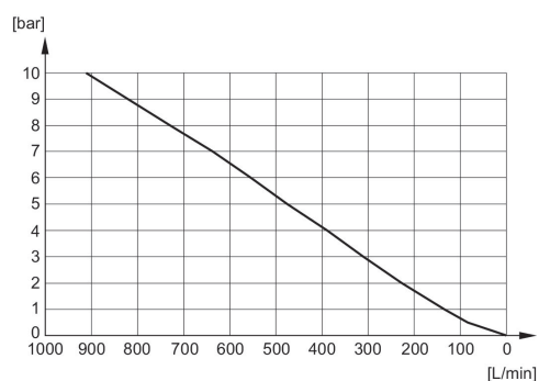
Durchflussdiagramm R414000155
