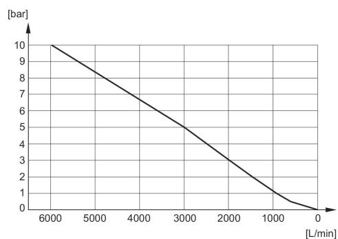
Durchflussdiagramm R412007877
