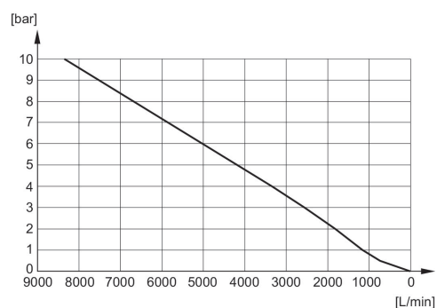
Durchflussdiagramm R412007878
