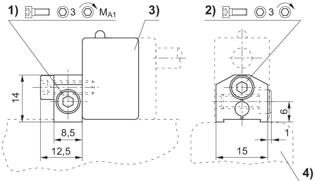
1) クランプねじ 2) センサー用固定ねじ 3) センサー 4) シリンダープロファイル
