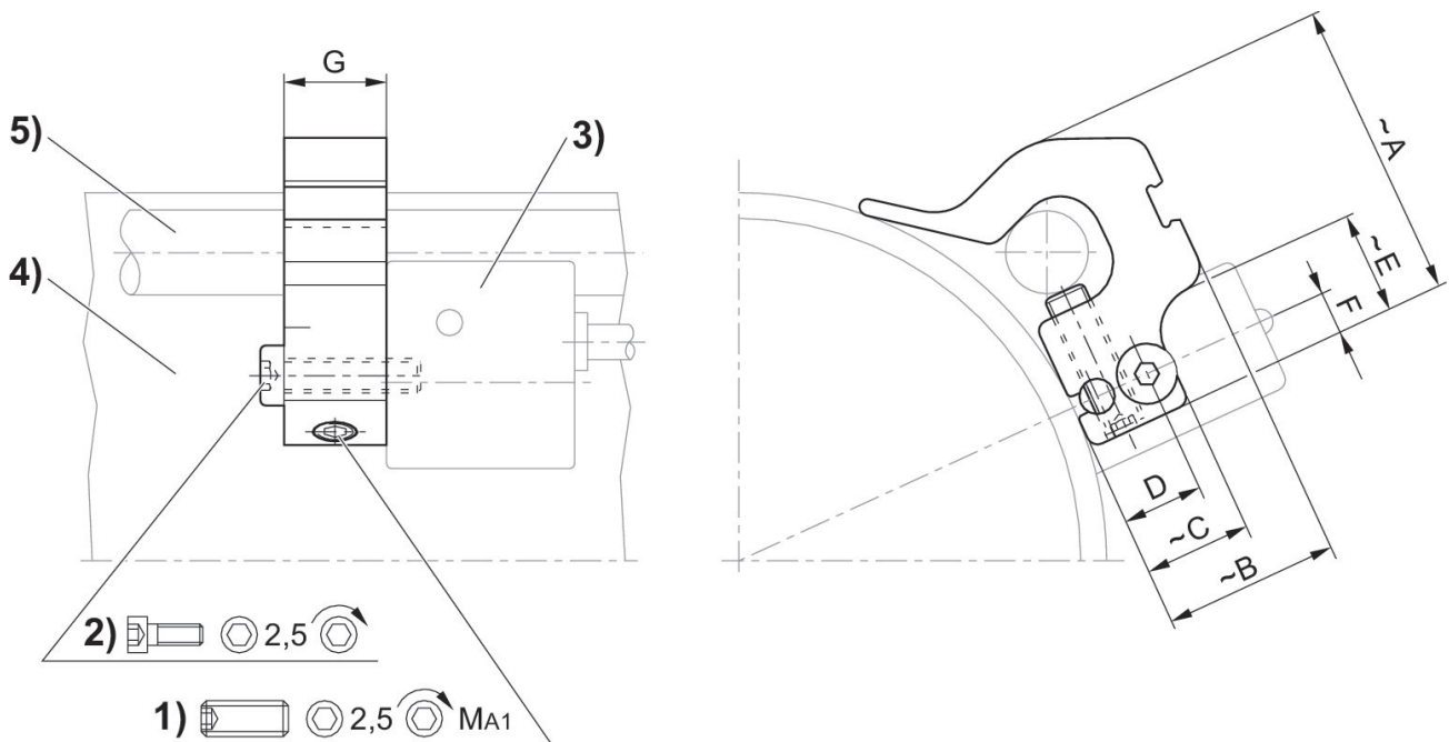
1) Klemmgewindestift 2) Befestigungsschraube für Sensor 3) Sensor 4) Zylinderprofil 5) Zuganker
