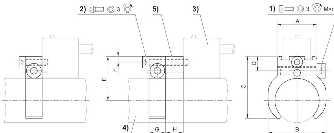
1) vite di bloccaggio 2) vite di fissaggio per sensore §) sensore 4) profilato cilindro 5) distanziale (se necessario)
