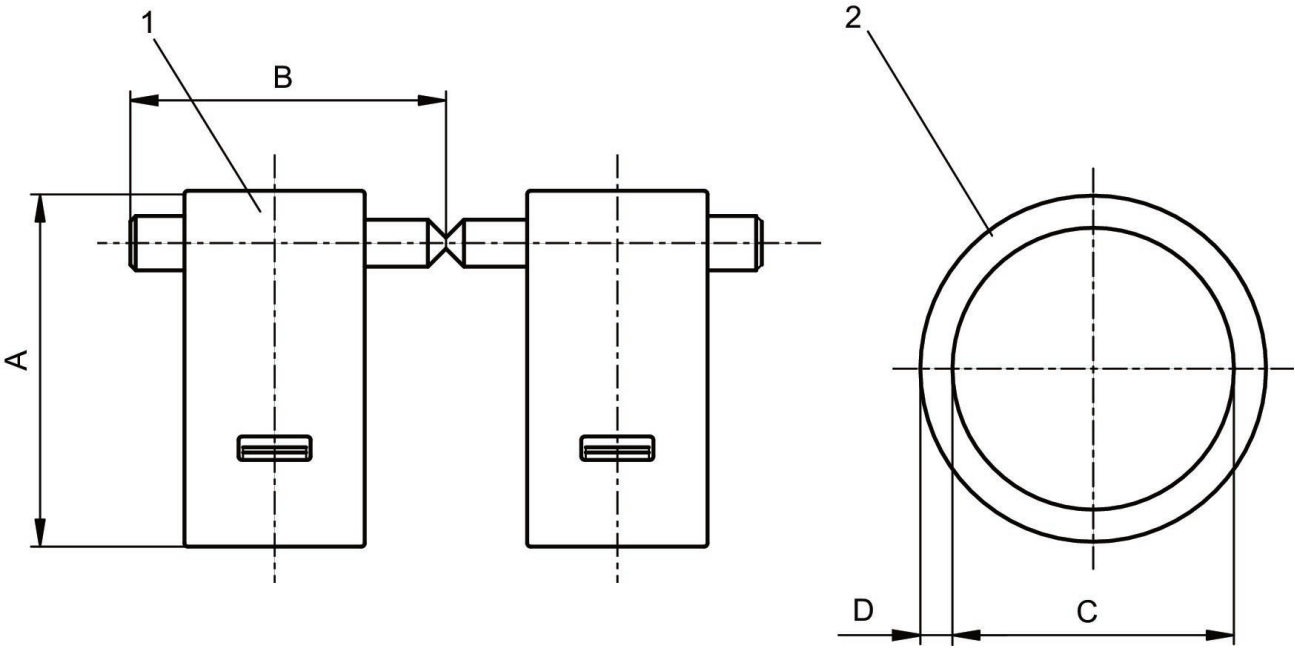
1) Koppelklammer 2) O-Ring
