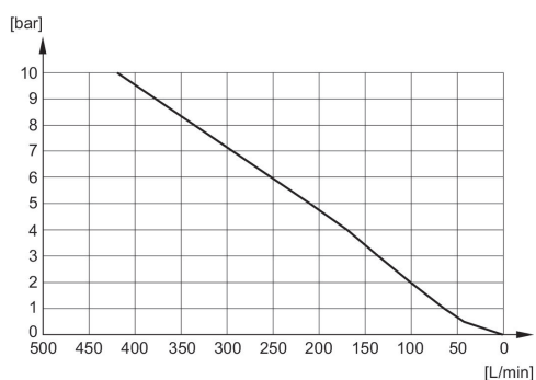
Diagramme du débit 1827000032
