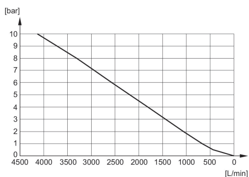
Diagramme du débit 1827000035
