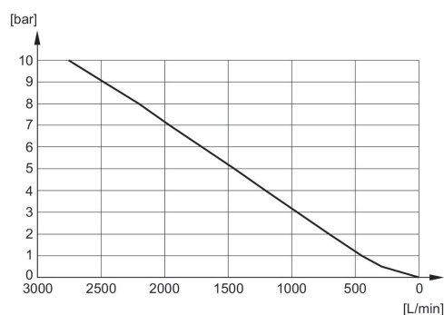
Diagramme du débit 1827000034
