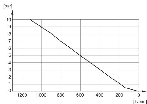
Diagramme du débit 1827000031
