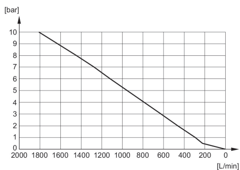
Diagramme du débit 1827000033
