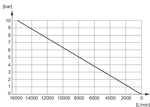
Durchflusssdiagramm 8145001000
