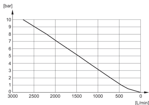
Durchflusssdiagramm 1827000034
