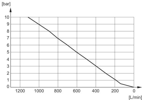
Durchflussdiagramm 1827000031
