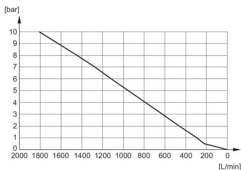
Durchflusssdiagramm 1827000033
