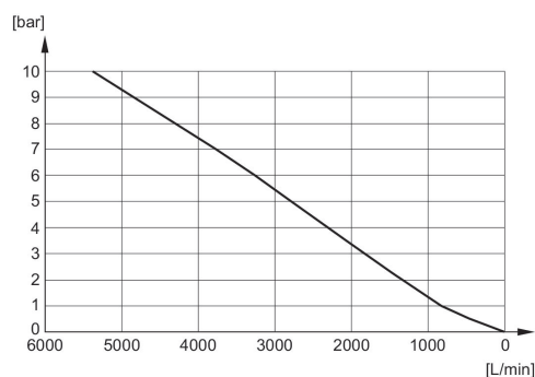
Durchflusssdiagramm 8145003400
