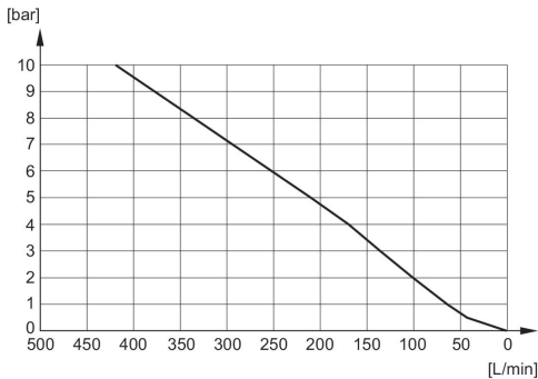
Durchflussdiagramm 1827000032
