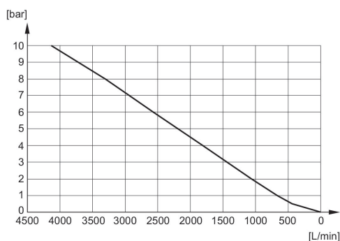
Durchflusssdiagramm 1827000035
