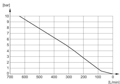
Diagramme du débit 1827000018
