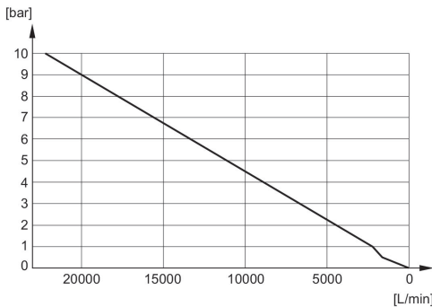
Diagramme du débit 1827000024
