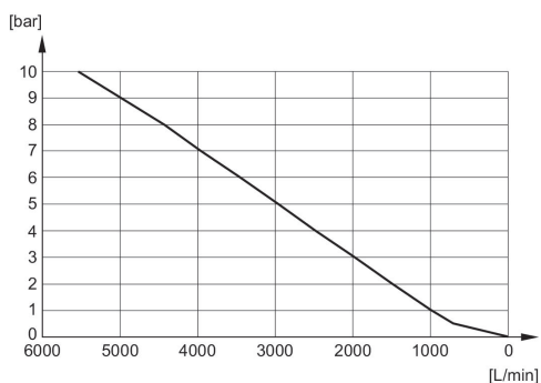
Durchflussdiagramm 1827000020
