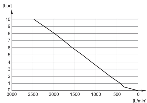
Durchflussdiagramm 1827000019
