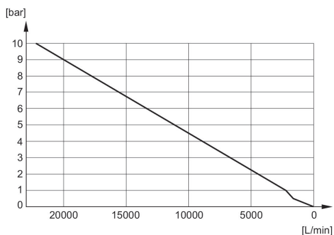
Durchflussdiagramm 1827000024
