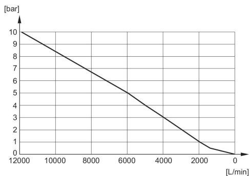
Durchflussdiagramm 1827000022
