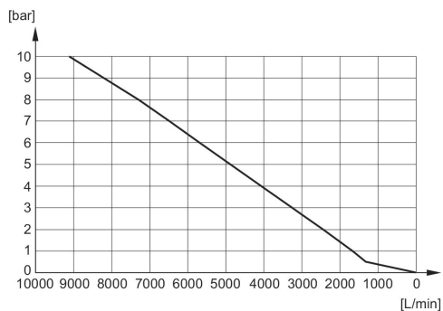
Durchflussdiagramm 1827000021
