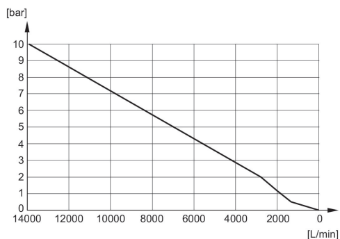
Durchflussdiagramm 1827000023
