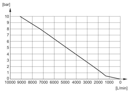
Durchflussdiagramm 1827000021
