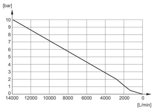
Durchflussdiagramm 1827000023
