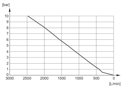
Durchflussdiagramm 1827000019
