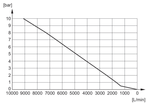
Durchflussdiagramm 1827000021
