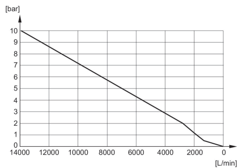
Durchflussdiagramm 1827000023
