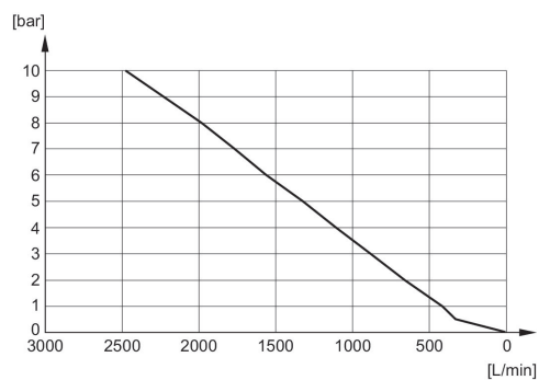
Durchflussdiagramm 1827000019
