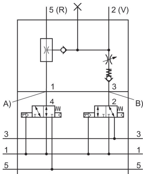
Fig. 5 ECV-HF03-...mit NO-Ansteuerung
