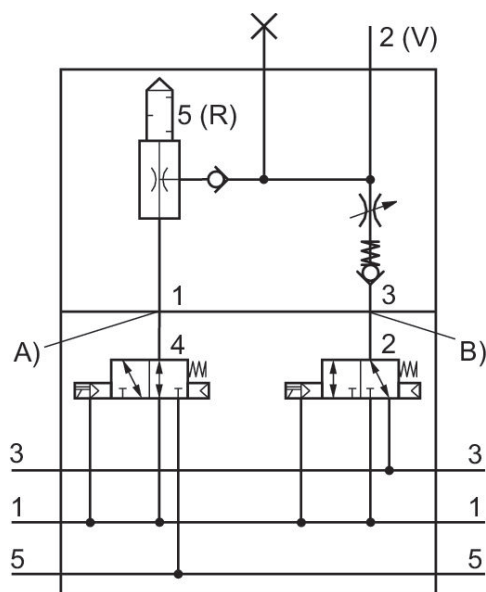
Fig. 7 ECV-HF03-...mit NO-Ansteuerung
