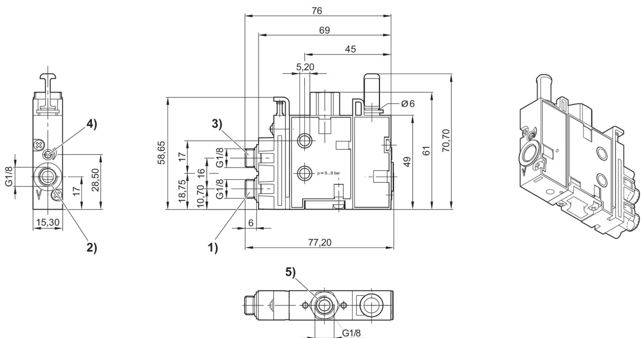
Fig. 3 ECV-PC-15-NN mit Entlüftungsanschluss
