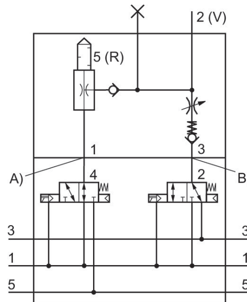
Fig. 7 ECV-HF03-...mit NO-Ansteuerung
