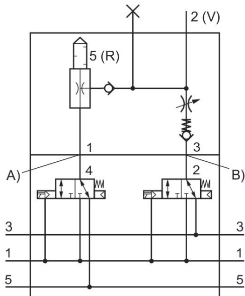
Fig. 8 ECV-HF03-...mit NC-Ansteuerung
