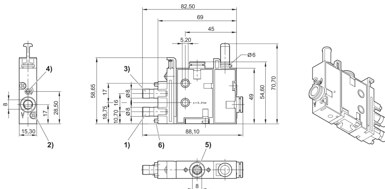
Fig. 1 ECV-PC-15-NN mit Entlüftungsanschluss
